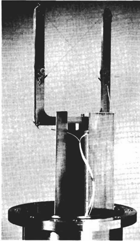
Fig. 4. Single Wire SEM
