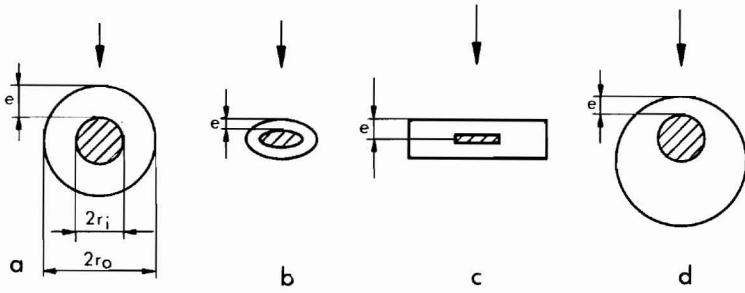
Fig. 1 : 50 Ω lines (a) Normal, (b) Elliptical, (c) Strip, (d) Eccentric
