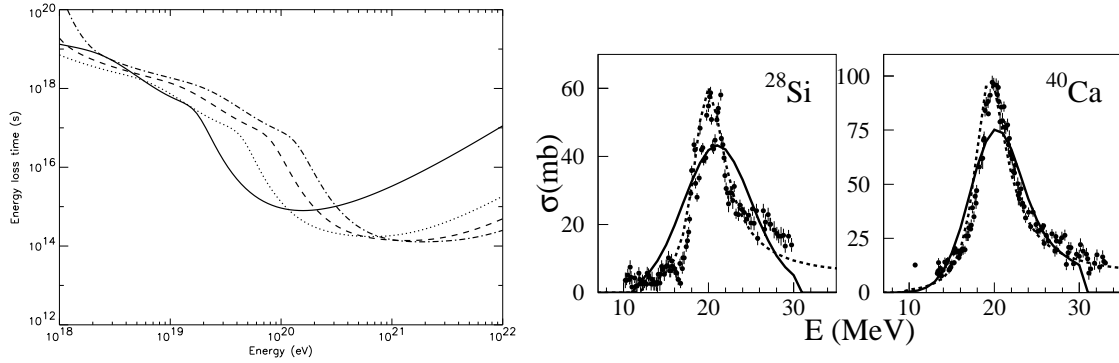
FIG. 4.8 : Gauche : Temps de perte d'énergie pour la photodésintégration (seule) sur le CMB et le CIB [84]; dans l'ordre en commençant par la ligne continue : He, C, Si et Fe. Droite : Sections efficaces de photoabsorption du Si et du Ca. Les données expérimentales sont comparées aux paramétrisations de [83] (lignes continues) et de [85] (tirets).
