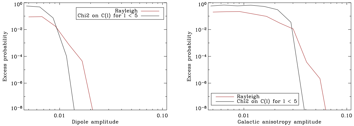
FIG. 3.4 : Sensibilité des méthodes de Rayleigh et des C_\ell à des anisotropies à grande échelle, en fonction de l'amplitude de ces anisotropies, pour 300 000 événements observés et une couverture de type « Auger - basse énergie ». Gauche : dipôle d'orientation aléatoire. Droite : excès gaussien vers le centre galactique, de dimensions \Delta\ell = 50^\circ et \Delta b = 10^\circ .
