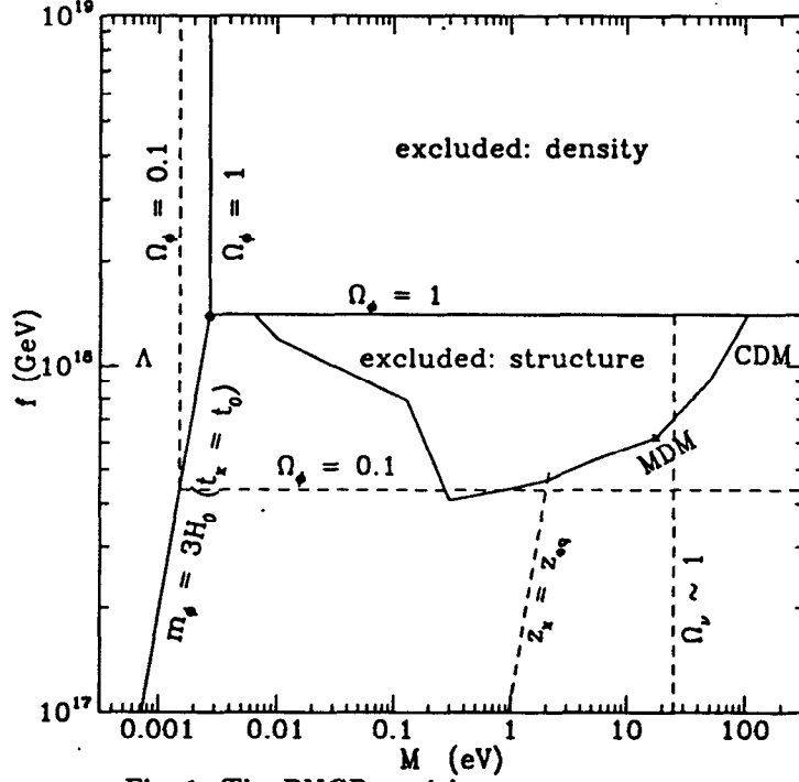
Fig. 1: The PNGB model parameter space.
