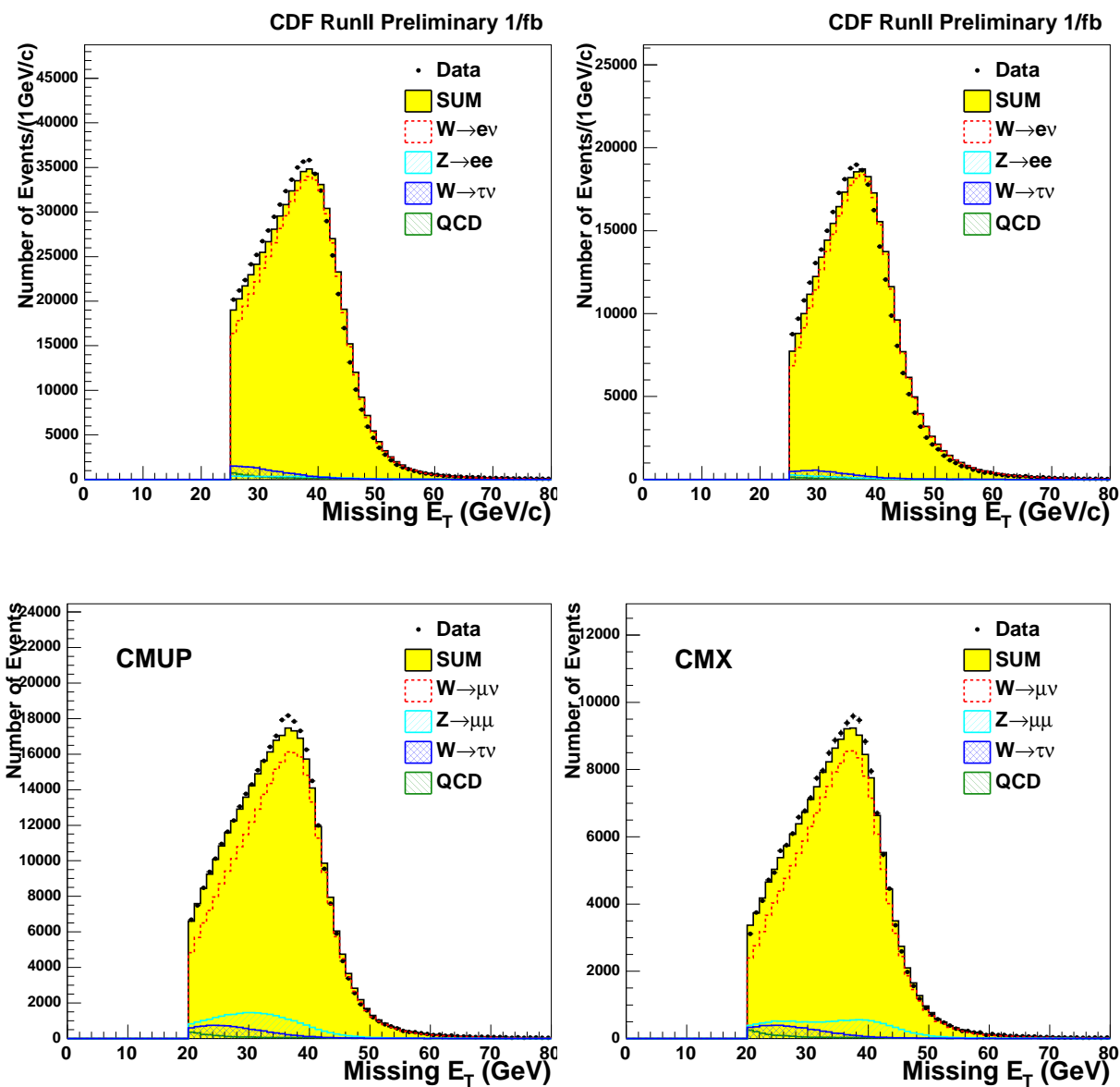
Figure 3.13: \cancel{E}_T distribution. Upper Left : Central Electron. Upper Right : Plug Electron. Lower Left : CMUP Muon. Lower Right : CMX Muon.
