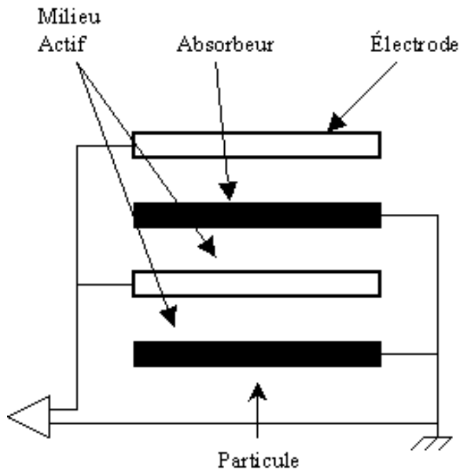
FIG. 3.6: Principe d'un calorimètre à segmentation. Des couches de matériaux denses sont interposées entre des couches de matériaux dits actifs. Ce sont ces dernières qui fournissent le signal récupéré par le système de lecture.
