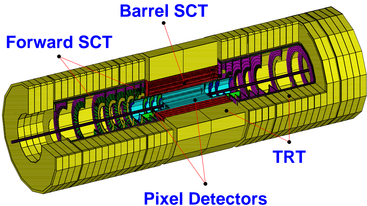
FIG. 2.10: Atlas, détecteur interne.
