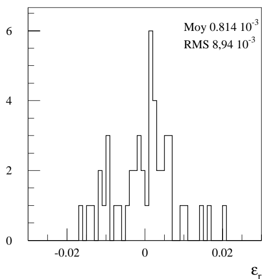
FIG. 3.16: Distribution des coefficients \varepsilon_r^k injectés pour simuler l'évolution des \alpha^k dans le cas de 48 zones. Ici la variance de ces coefficients est de 1%.
