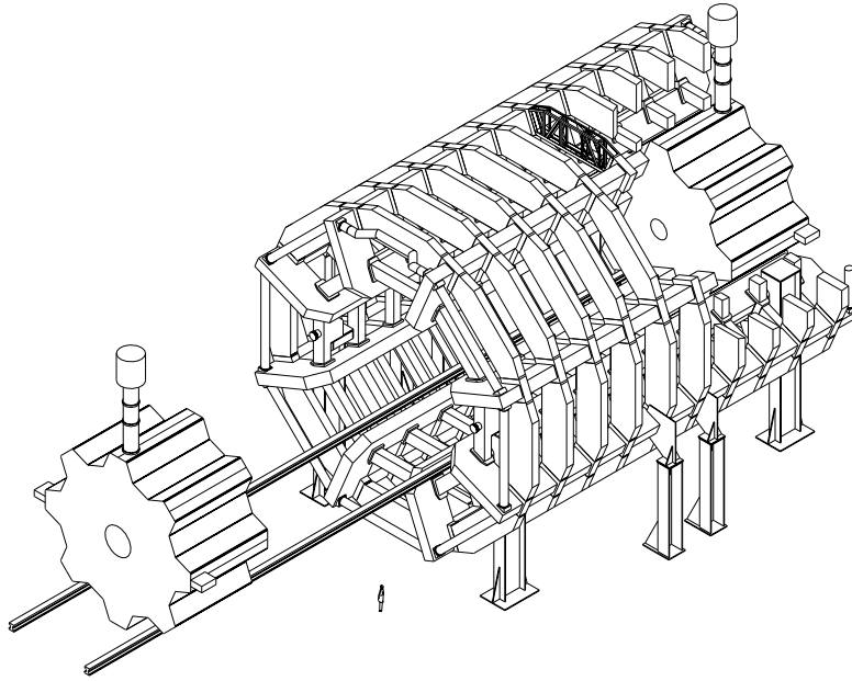
FIG. 2.16: Vue tridimensionnelle du système de bobines produisant le champ toroïdal pour le spectromètre à muons d'ATLAS.
