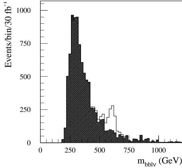
FIG. 4.13: Distribution de la masse invariante de bbl\nu après coupures. En noir, bruit de fond, en blanc bruit de fond + signal. Le signal représenté ici est le cas de la production d'un \tilde{s} -quark de 600 GeV et de largeur 0.5 GeV. Normalisation pour 3 années au LHC à basse luminosité.
