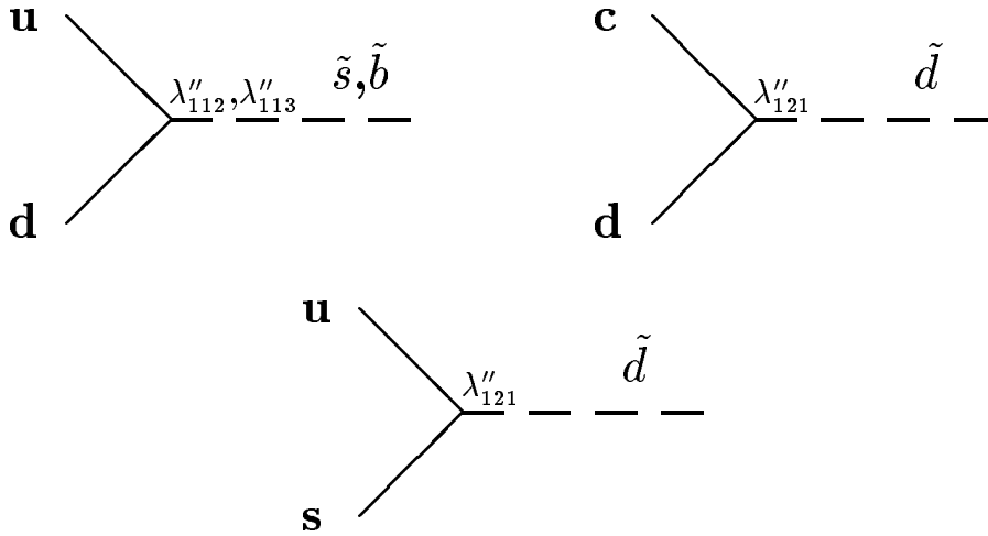
FIG. 1.6: Exemples de production de squarks par R-parité violée dans des collisionneurs proton-proton. Ici on n'a considéré que les cas où au moins un des quarks initiaux était un quark de valence du proton.
