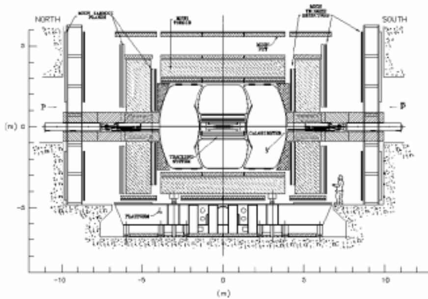
FIG. 2.19: Vue d'ensemble du détecteur à muons de D\emptyset .
