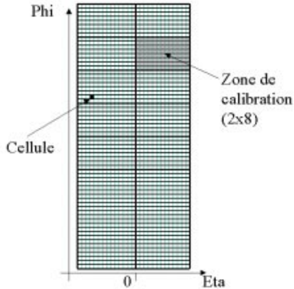
FIG. 3.11: Exemple de découpage du calorimètre électromagnétique (ici la partie centrale) en zones de calibration. Dans le cas présent, il s'agit d'un découpage en 48 zones. La partie centrale du calorimètre est alors divisée en deux parties égales suivant \eta et en huit parties suivant l'angle azimutal \phi . Une des zones est grisée afin d'avoir un ordre de grandeur de la taille relative de celles-ci avec la taille d'une cellule du calorimètre (ici, granularité de 0,1 \times 0,1 ).
