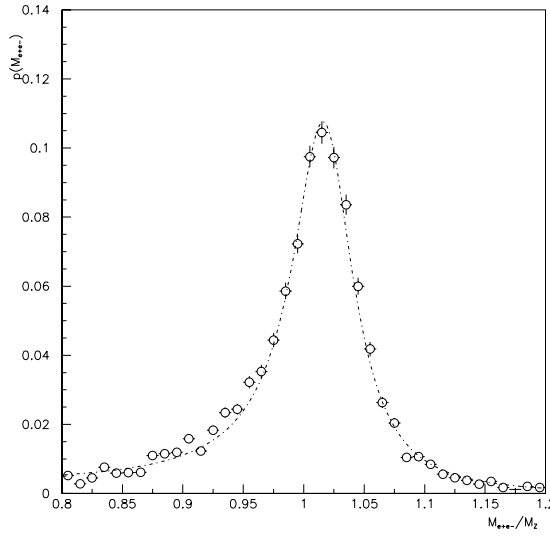
FIG. 3.15: Distribution de la masse invariante reconstruite des paires e^+e^- provenant de la désintégration du Z par le processus de Drell-Yan (cercles). La courbe est la fonction analytique utilisée dans l'algorithme.
