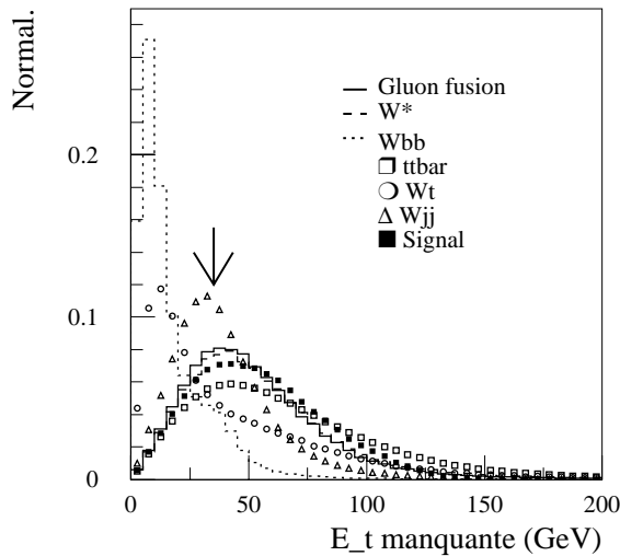
FIG. 4.7: Distribution de l'énergie transverse manquante. Le signal représenté ici correspond à la production d'un \tilde{s} -quark de masse 300 GeV et de largeur 0.5 GeV. La somme des événements a été normalisée à 1.
