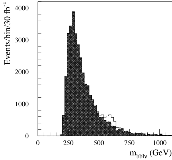
FIG. 4.11: Distribution de la masse invariante lbb pour le bruit de fond (en noir) et le bruit de fond + signal (blanc) après trois années à basse luminosité au LHC pour un \tilde{s} -quark de masse 600 GeV et de largeur 0.5 GeV.
