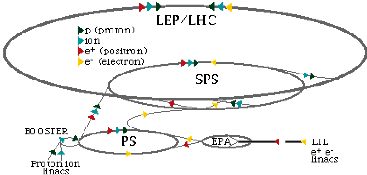
FIG. 2.4: Le système d'injection au LHC. Les protons seront accélérés dans le LINAC puis dans le booster jusqu'au Proton Synchrotron (PS), où leur énergie passera de 1,4 à 25 GeV. Le Super Proton Synchrotron (SPS) les amènera jusqu'à 450 GeV avant de les injecter dans l'anneau du LHC, où leur énergie finale sera de 7 TeV.
