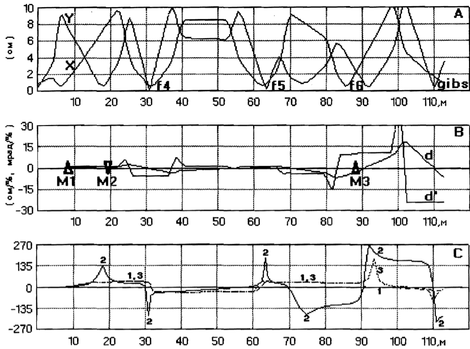
Рис. 4. Основные функции для режима с усиленным импульсным разрешением. А, В - линейные отгибающие пучка, линейная и угловая дисперсии. С - Разрешающая способность (отношение линейной дисперсии к эталонной линейной отгибающей, см. в тексте): 1 - стандартный режим, 2,3 - варианты режимов с усиленным импульсным разрешением
