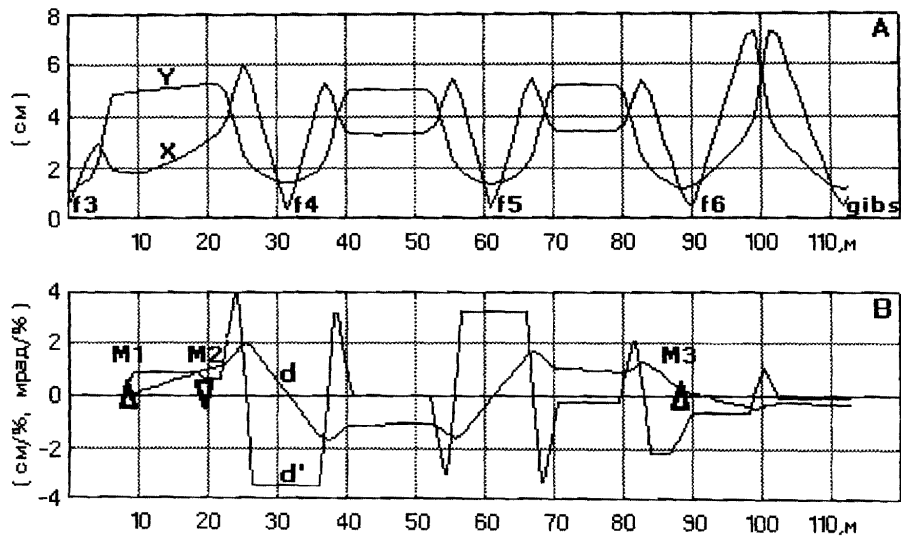
Рис. 2. Основные функции для стандартного режима каналов VP-1 и 6V. А - Линейные огибающие пучка ( 2\sigma ) в горизонтальной (X) и вертикальной (Y) плоскостях ( \epsilon_x \simeq \epsilon_y = 40\pi мм · мрад, \delta_p = 0 ). В - Линейная и угловая дисперсии
