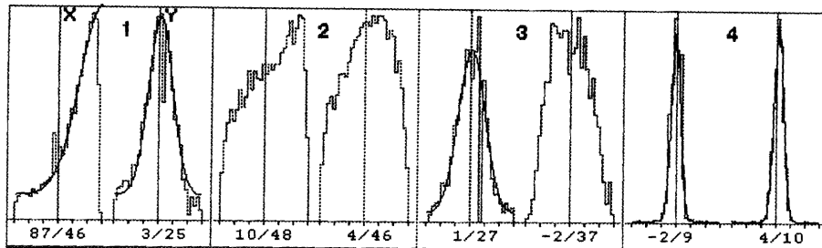
Рис. 3. Формирование пучка трития: координатные распределения в горизонтальной (X) и вертикальной (Y) плоскостях при P_{3H} = 6 \text{ ГэВ/с} . 1 - после магнита M1 ("хвост" первичного пучка \alpha -частиц), 2 - на входе в дублет D1, 3 - на входе в дублет D3, 4 - в фокусе F6. Цифры под гистограммами: среднее значение/среднеквадратичное отклонение, мм. Диапазон горизонтальной шкалы - \pm 90 мм, гладкие кривые - аппроксимация гауссианом
