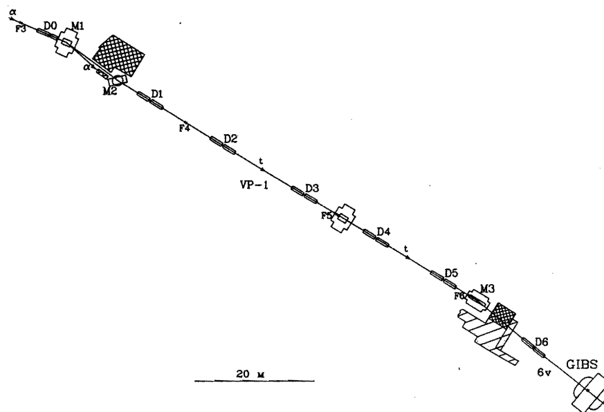
Рис. 1. План магнитооптического канала для формирования пучка трития на установке ГИБС. \alpha - трасса первичного пучка {}^4\text{He} , D0...D7 - дублиты квадрупольных линз, M1, M2, M3 - поворотные магниты
