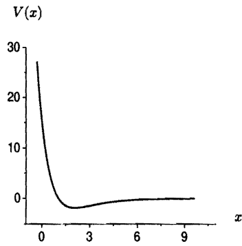
Рис. 1. Вид потенциала Морзе V(x) с параметрами M=8.876 , D=0.104 , \alpha=0.67 , x_\alpha=2.09
