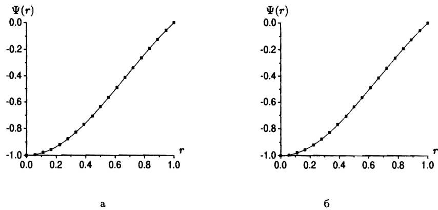
Рис. 3. Вид функции \Psi(r) при b_0 = \pi и а) k=1.E-2 , б) k=1.E-5 . Сплошная линия - расчет по формуле (71), пунктирная линия - численный результат
