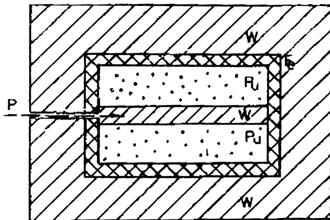
Рис. 1. Цилиндрическая плутониевая сборка с вольфрамовой мишенью диаметром 3 см и длиной 14 см, плутониевым бланкетом диаметром 7,2 см, стальным и вольфрамовым рефлексорами с толщинами, соответственно, 2,4 и 10 см. Плутониевые стержни имеют танталовую и стальную оболочки толщиной 0,1 и 0,3 мм. Пучок ускоренных протонов вводится в вольфрамовую мишень через осевую щель на глубину 1 см
