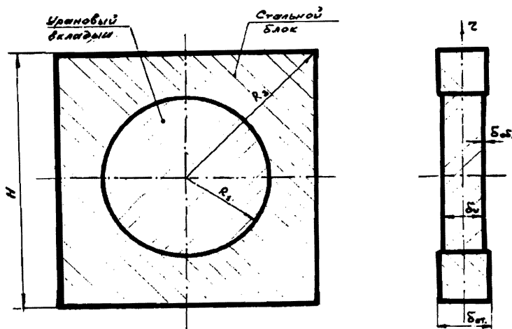
Рис. 4. Размер вставки H = 170 мм, ее толщина \delta_{ст} = 31 мм. Толщина (U – Мо)– вкладыша \delta_v = 25 мм. Толщина его оболочки \delta_{об} = 2,5 мм. Радиус вкладыша по урану R_1 = 53 мм ( R_2 = 120 мм)
