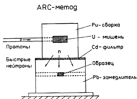
Рис. 5. Принципиальная схема экспериментальной реализации ARC-метода
