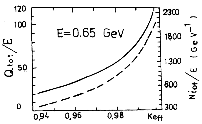
Рис.3. Зависимость тепловыделения (сплошная кривая) и выхода нейтронов (пунктир) от коэффициента мультипликации при E = 0,66 ГэВ
