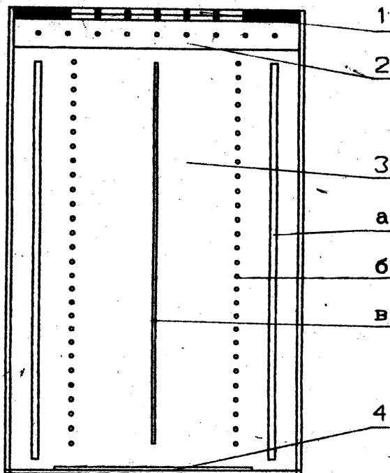
Рис.2. Схематическое устройство телескопа-спектрометра: 1 - входное окно с двумя опорными сетками 2 - многонитяной пропорциональный счетчик 3 - ионизационная камера: а) анод; б) сетка; в) катод
