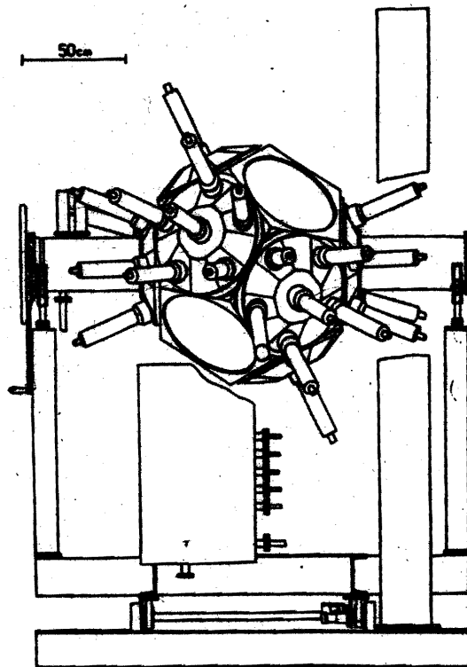
Рис. 1. Общий вид установки ФАЗА
