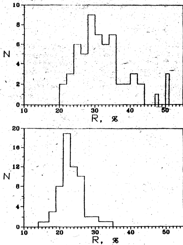
Рис.5. Распределения сцинтилляторов по амплитудному разрешению для \alpha -частиц из ^{214}\text{Am} . Вверху - для сплошных световодов, внизу - для комбинированных световодов новой конструкции
