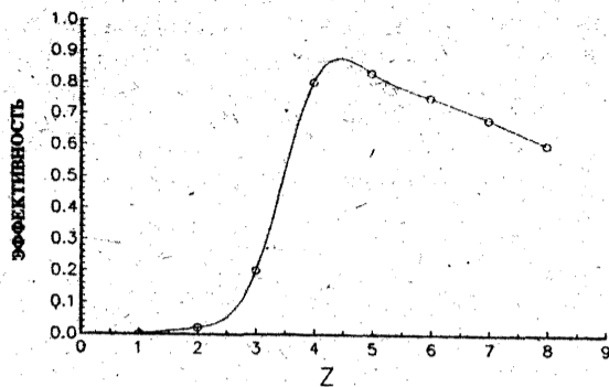
Рис.7. Расчетная зависимость эффективности регистрации фрагментов с зарядом Z сцинтилятором толщиной 20 мг/см
