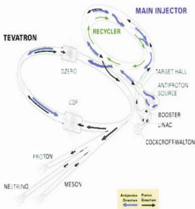
Figura 2.1: Schema del collisionatore Tevatron e dei preacceleratori booster e main injector, e della sorgente di antiprotoni includente il recycler.
