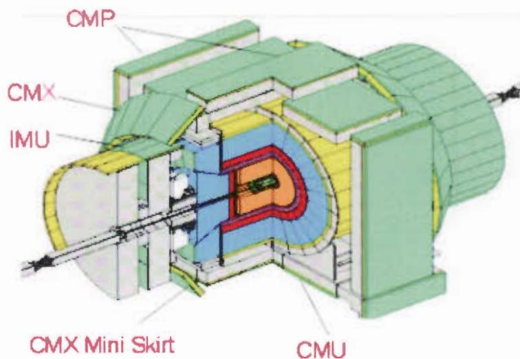
Figura 2.5: Disposizione dei rivelatori esterni di muoni
