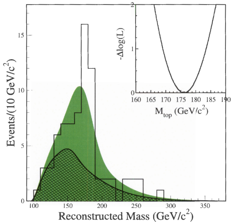
Figura 1.1: Eventi del campione single lepton come getti taggati b ricostruiti nell'ipotesi t\bar{t} . Area verde tratteggiata: contributo del fondo. Area verde oscurata: distribuzione attesa per segnale+fondo alla massa scelta dal fit. Istogramma: dati sperimentali. L'inserito mostra l'andamento del \chi^2 del fit in funzione di M_{top} .
