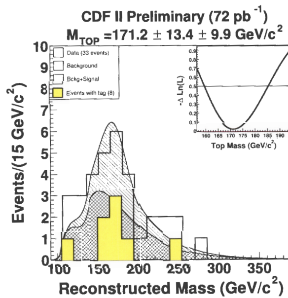
Figura 4.2: Fit a due componenti della distribuzione di massa del top ottenuto dalla analisi degli “eventi duri” (Marzo 2003).
