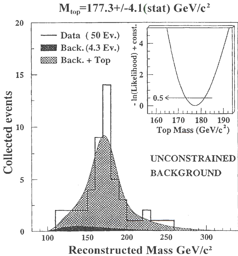
Figura 3.2: Massa del top ottenuta dal fit degli eventi puliti nel RunI.
