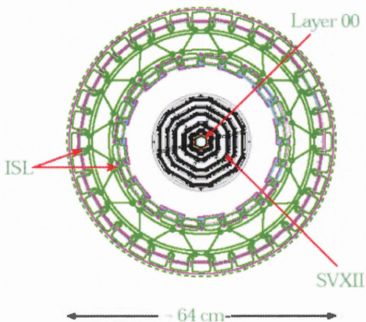
Figura 2.3: Sezione centrale del tracciatore a silicio di CDF2
