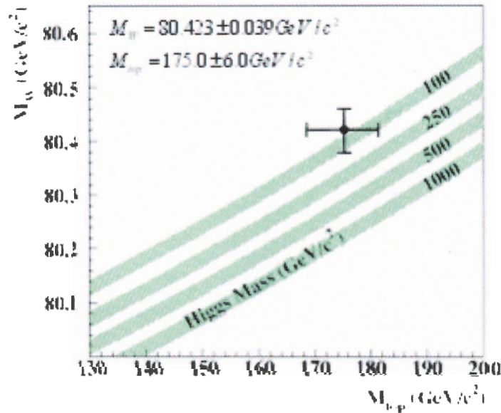
Figura 1: Correlazione attesa nel Modello Standard fra M_{top} e M_W in funzione della massa del bosone di Higgs (bande ombreggiate). Il punto con le bande di errore indica le misure attualmente disponibili (primavera 2003) della massa del top e del W.
