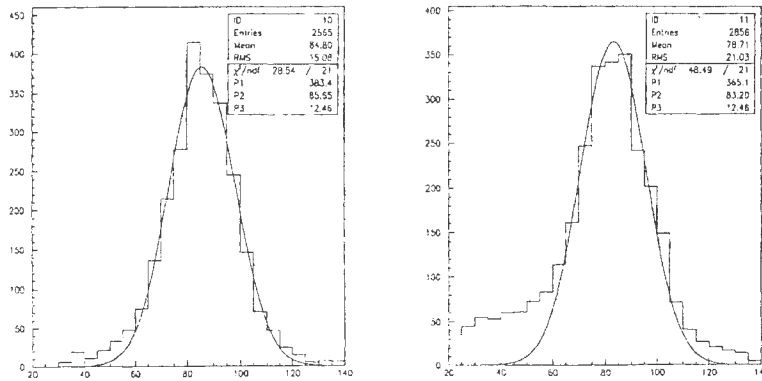
Figura 3.1: Massa delle coppie dei getti attribuiti al decadimento del W nel campione single-lepton pre-tag del RuI. a)Eventi puliti, b)intero campione.
