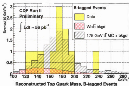
Figura 5.1: Distribuzione di massa da eventi con b-tag
