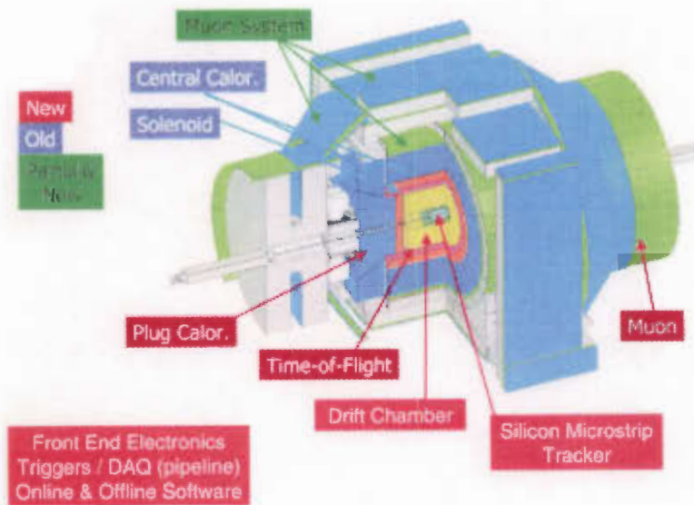
Figura 2.2: Presentazione del rivelatore CDF2
