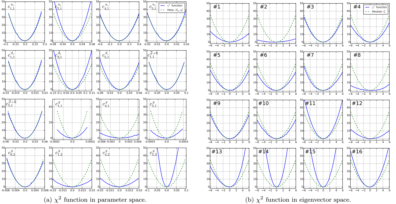
(a) \chi^2 function in parameter space.
