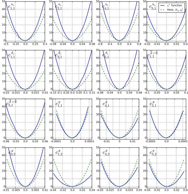
(a) \chi^2 function in parameter space.
